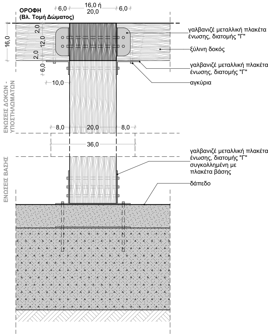
ΣΚΕΛΕΤΟΣ ΑΝΑΨΥΚΤΗΡΙΟΥ ΥΠΟΣΤΥΛΩΜΑΤΑ - ΔΟΚΟΙ ΤΥΠΙΚΗ ΤΟΜΗ
