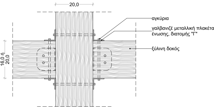
ΣΚΕΛΕΤΟΣ ΑΝΑΨΥΚΤΗΡΙΟΥ ΥΠΟΣΤΥΛΩΜΑΤΑ - ΔΟΚΟΙ ΤΥΠΙΚΗ ΚΑΤΟΨΗ
