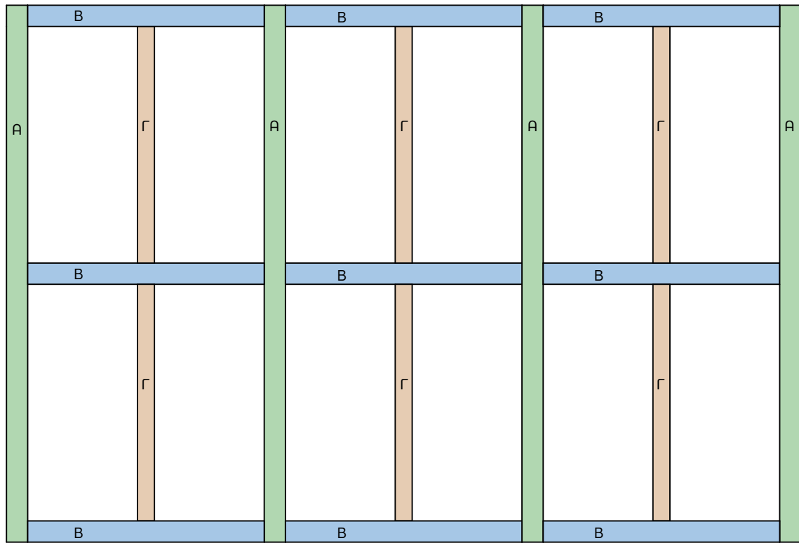
ΔΟΚΟΙ ΟΡΟΦΗΣ ΑΝΑΨΥΚΤΗΡΙΟΥ (ΚΛΙΜΑΚΑ 1:50)
