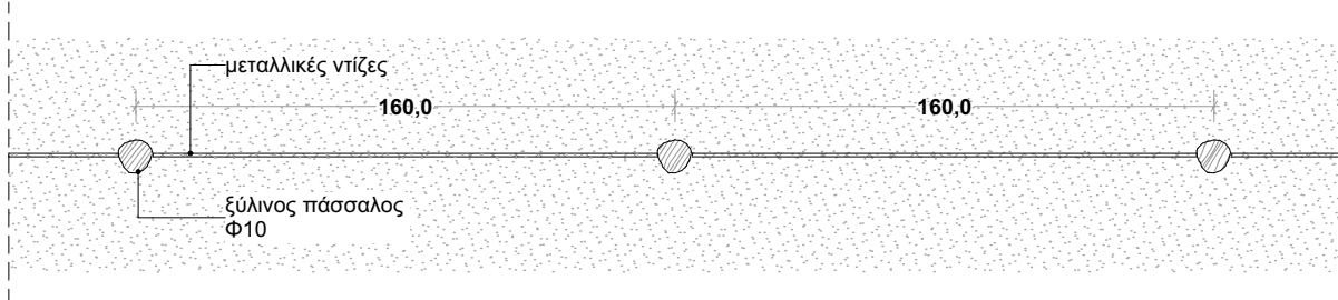
ΣΤ1: ΠΕΡΙΦΡΑΞΗ ΑΣΦΑΛΕΙΑΣ ΚΑΤΩΨΗ
