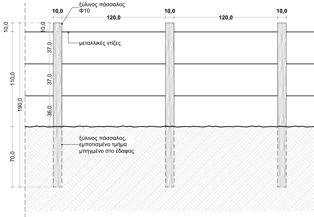
ΣΤ1: ΠΕΡΙΦΡΑΞΗ ΑΣΦΑΛΕΙΑΣ ΟΥΨΗ
