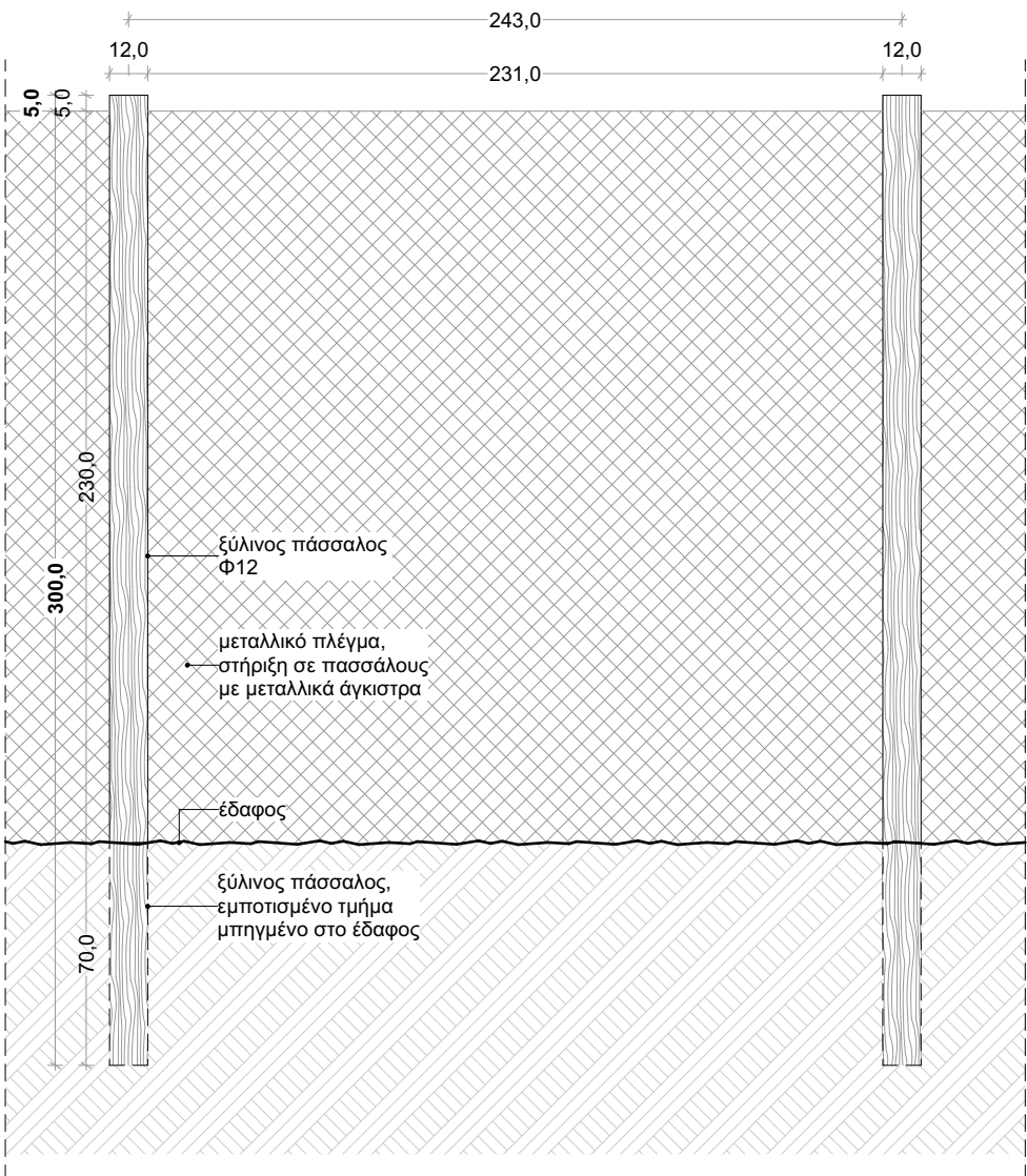
ΠΦ1: ΜΕΤΑΛΛΙΚΗ ΠΕΡΙΦΡΑΞΗ ΕΞΩΤ. ΟΥΨΗ
